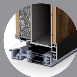
Aluminium- Bodenschwelle
