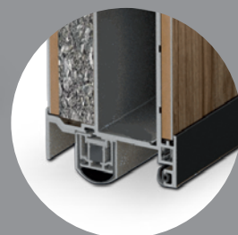
Absenkbare Bodendichtung ohne Schwelle
